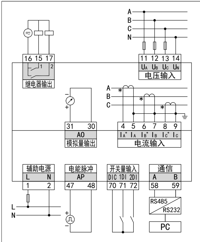
PD194Z-AHY 接线端子图：
